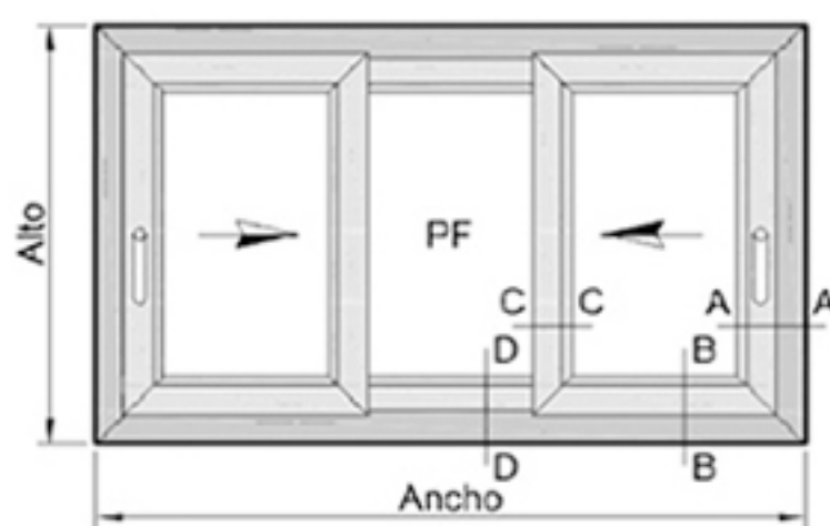
Puerta de 2 guías y 2 hojas móviles con 1 paño fijo central
