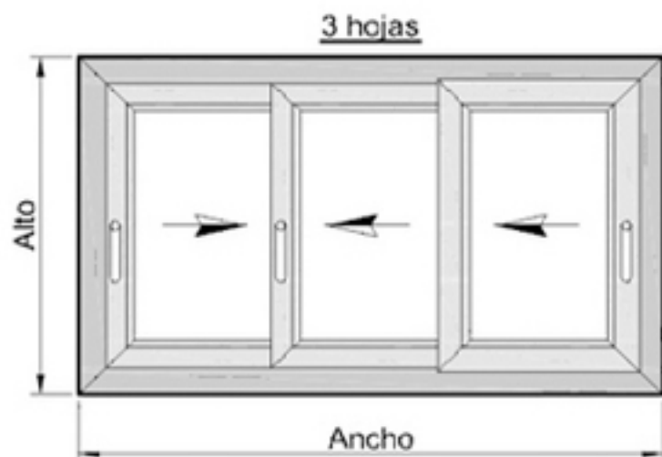
Puerta de 3 guías y 3 hojas móviles
