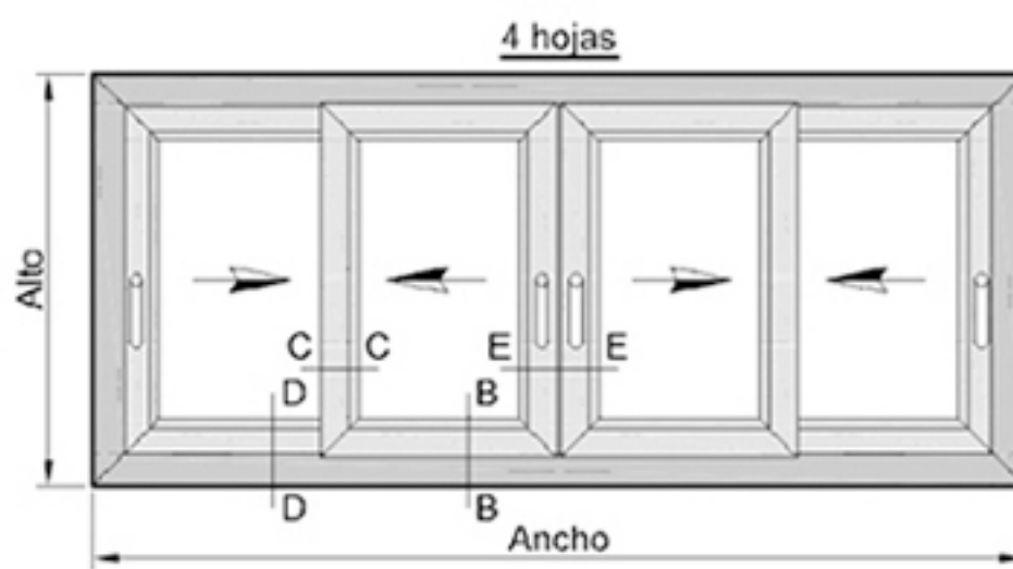
Puerta de 2 guías y 4 hojas móviles
