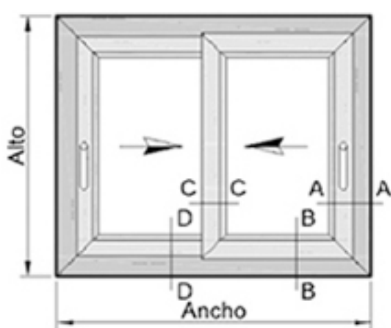
Puerta de 2 guías y 2 hojas móviles
